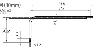
深孔2倍 *2
