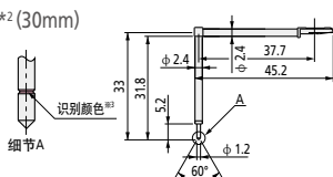
深槽用 *2(30mm)
