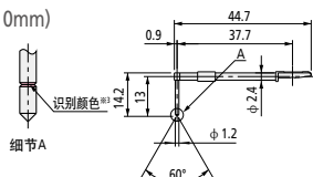
深槽用 *2(20mm)
